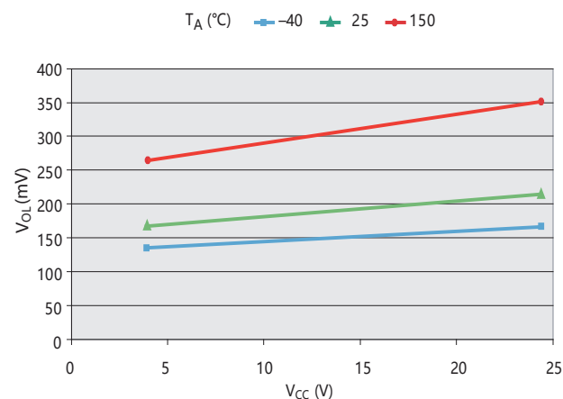
低电平(输出导通) VS 工作电压
